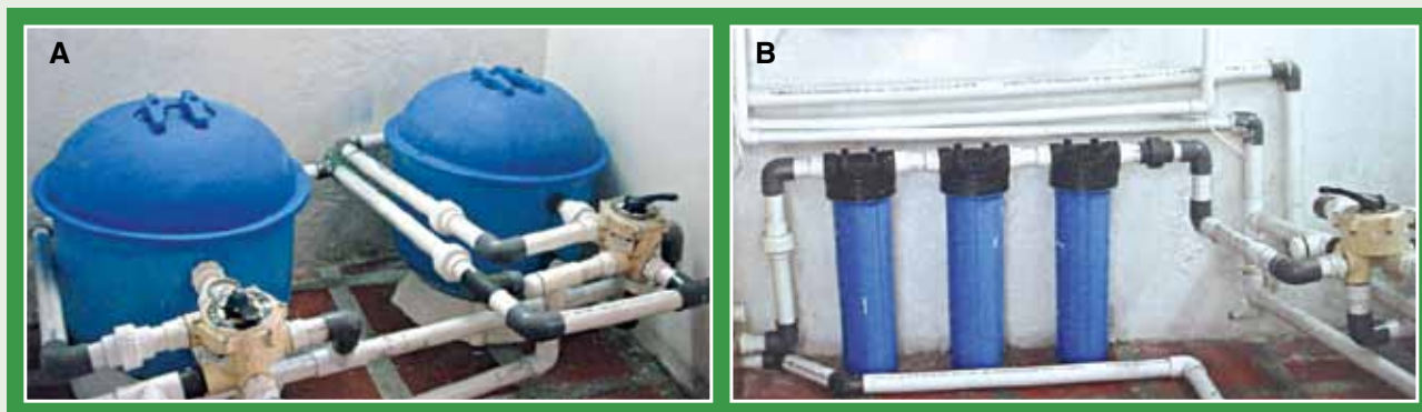
Figura 9. Sistema de filtración del LABBIP. Filtros de arena (A) y de cartucho (B).
