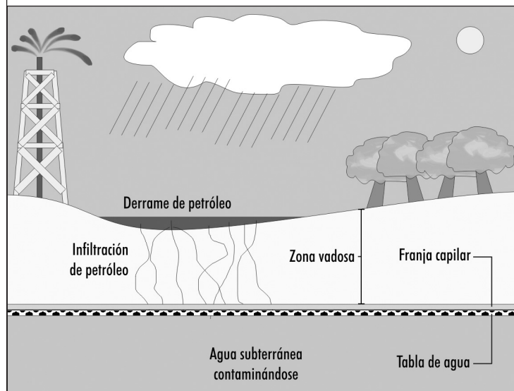
Figura 9. Contaminación de agua subterránea por infiltración de petróleo. Modificado de: Idaho museum natural history, 2002.
