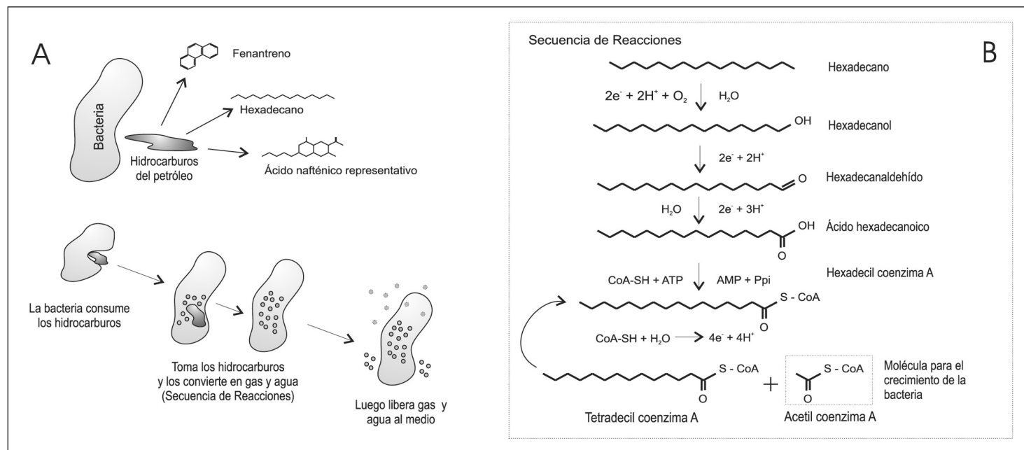
Figura 13. A. Diagrama de la biodegradación de hidrocarburos de petróleo. Modificado de: Environmental Protection Agency, 2001. B. Secuencia abreviada de la biodegradación del hexadecano realizada por Pseudomonas oleovorans . Fuente: Prince, 2002
