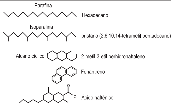
Figura 12. Estructuras químicas de algunos de los hidrocarburos que conforman el petróleo. Tomado de: Prince, 2002. En: Bitton, 2002.
