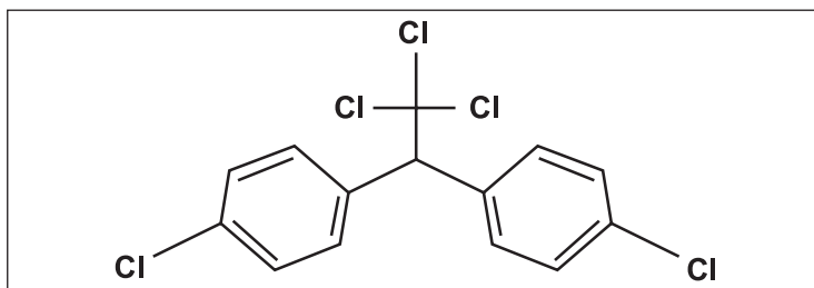
Figura 14. DDT (1,1,1-tricloro-2,2-di(p-clorofenil)etano). Tomado de: Prince, 2002.
