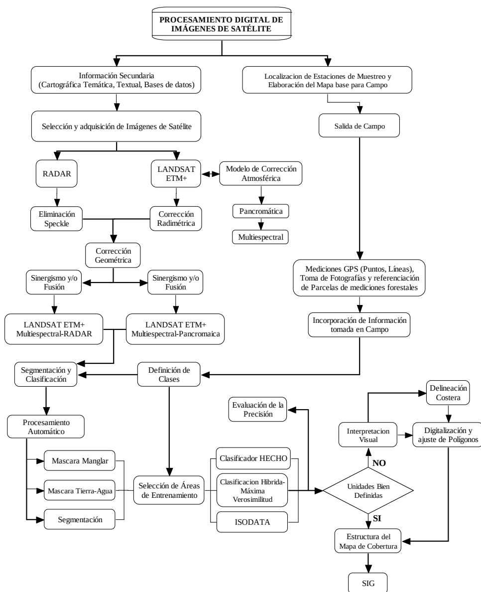
Figura III-4. Metodología de procesamiento digital de imágenes de satélite para generación de cartografía temática de cobertura de manglar.
