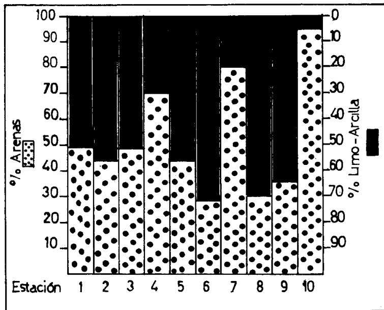
Figura 3. Granulometría del sedimento, realizada mediante el método de Bouyoucos (IGAC, 1979), y utilizando la nomenclatura propuesta por Vernette (1982); en la figura se representan los porcentajes de arena y de la fracción limo-arcilla determinados por el análisis en cada una de las muestras.
