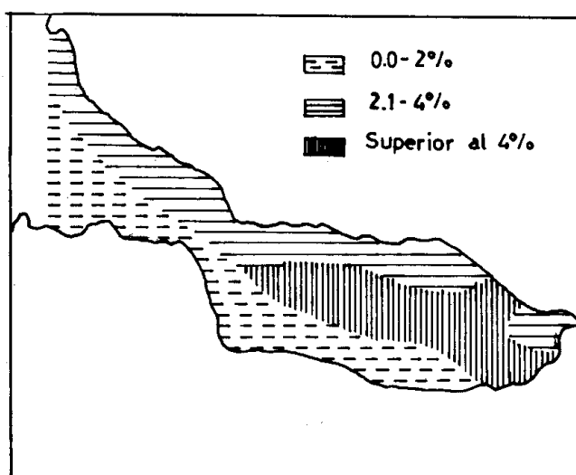
Figura 6. Distribución de la materia orgánica. Tomando 3 intervalos según el contenido de materia orgánica particulada, los porcentajes son representados en un esquema de la ciénaga para facilitar la visualización de las zonas más o menos ricas en este recurso.
