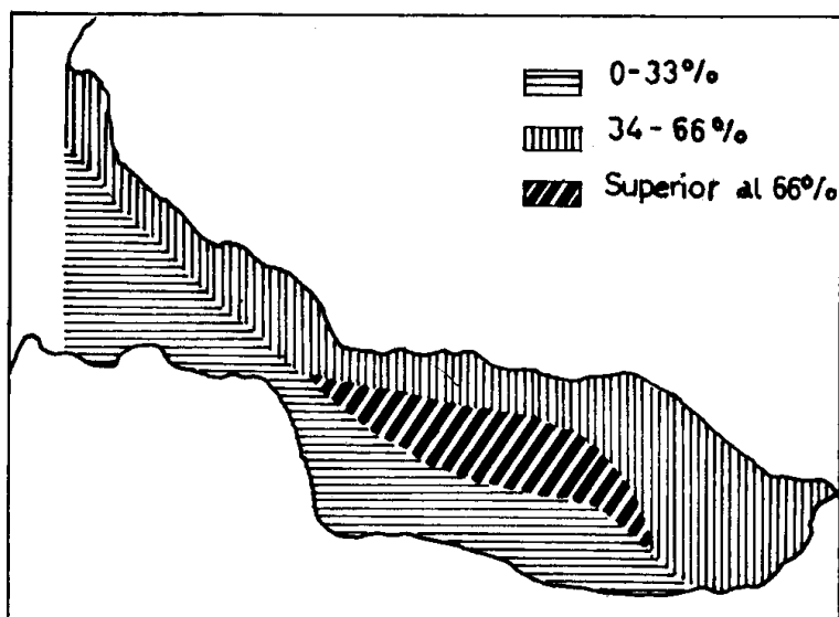
Figura 4. Distribución de la fracción limo-arcilla. Los valores de esta fracción determinados como se indicó en la figura anterior son representados en un esquema de la ciénaga tomando 3 intervalos de porcentajes.
