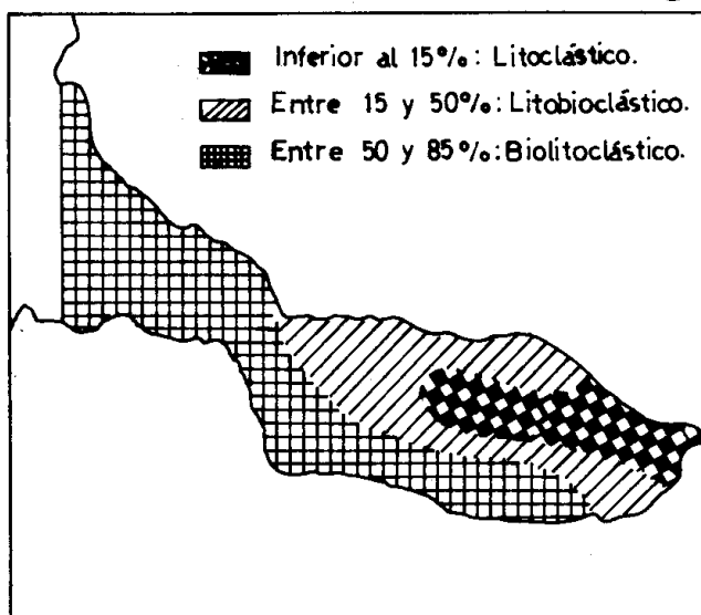
Figura 5. Distribución del carbonato de calcio, utilizando los intervalos y la nomenclatura correspondiente propuestos por Vernet (1982), se representaron en un esquema de la ciénaga.
