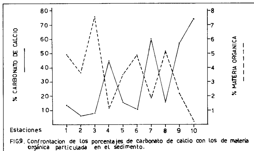
Figura 9. Confrontación de calcio y la materia orgánica particulada. Tomando los valores de carbonato de calcio y de materia orgánica particulada en cada estación, se graficaron simultáneamente con el fin de observar el comportamiento de los dos parámetros comparativamente, el cual demostró ser inverso.
