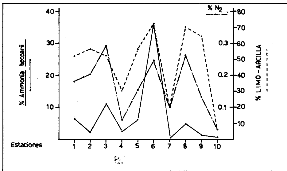
Figura 12. Confrontación de los porcentajes de nitrógeno, limo-arcilla e individuos de Ammonia beccarii . Graficando los valores de estos tres parámetros simultáneamente para cada una y todas las estaciones, se logró establecer que también existía una relación directa entre el número de especímenes de la biocenosis y el contenido de nitrógeno y limo-arcilla en el sedimento.
