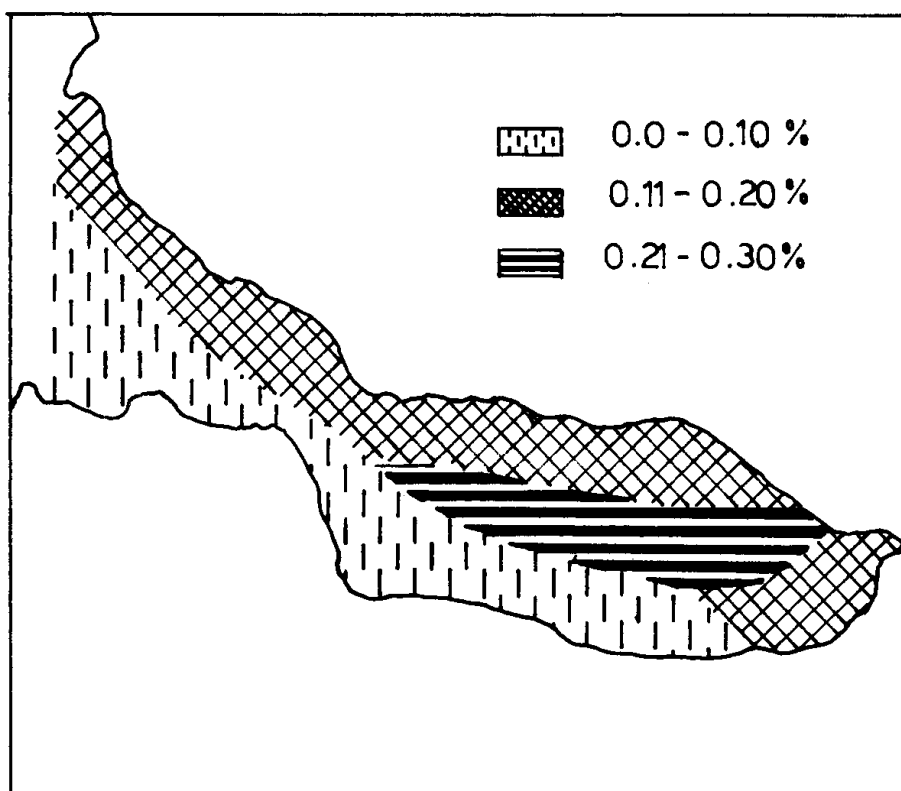
Figura 7. Distribución del nitrógeno orgánico. De la misma manera descrita para la figura anterior, se tomaron 3 intervalos correspondientes a diferentes contenidos de nitrógeno orgánico en el sedimento y se representaron en un esquema de la ciénaga, el cual muestra claramente qué zonas contienen mayores o menores porcentajes.
