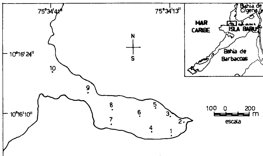
Figura 2. Delimitación del área de estudio. La ciénaga de los Vásquez se encuentra situada en el costado noroeste de isla Barú. Los puntos numerados corresponden a las estaciones donde se colectaron los sedimentos.
